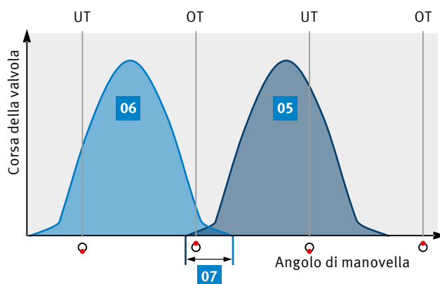
Sovrapposizione valvole
